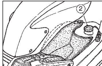
FIG. 13 1. Tapa compartimento bomba aceite 2. Depósito aceite
