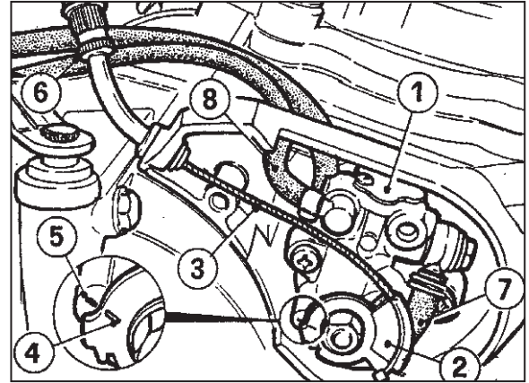
FIG. 14 POMPA OLIO 1. Pompa olio 2. Leva comando pompa 3. Cavo comando 4. Riferimento sulla leva 5. Riferimento corpo pompa 6. Registro pompa 7. Condotto aspirazione 8. Condotto di mandata
