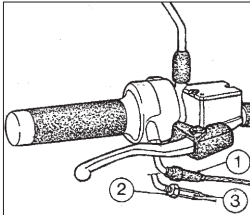
FIG. 15 1. Cappuccio 2. Controddado 3. Vite di registro 4. Vite fissaggio pannello
