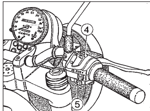
BILD 12 1. Kraftstoffhahn 2. Zündschlüssel 3. Starterhebel 4. Rechter Umschalter 5. MotoranlassKnopf (seite 53)
